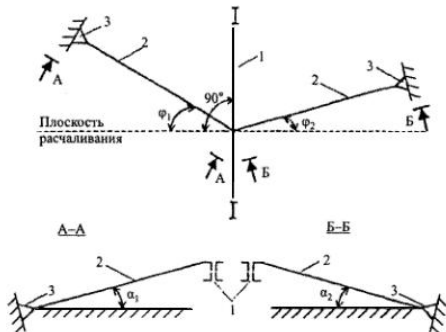
Рисунок К.2 - Схема раскрепления ферм расчалками
